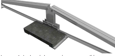
Ejemplo de contrapeso de hasta 400 mm de ancho sobre portalastre .
